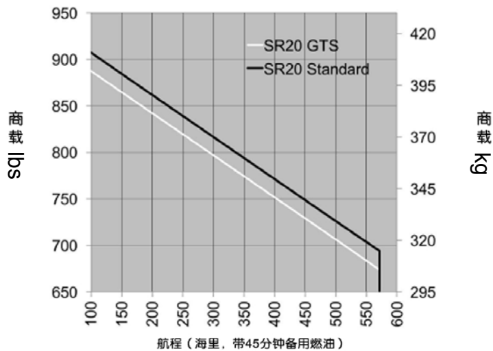
SR20 高速巡航@8,000英尺 (155KTAS)
